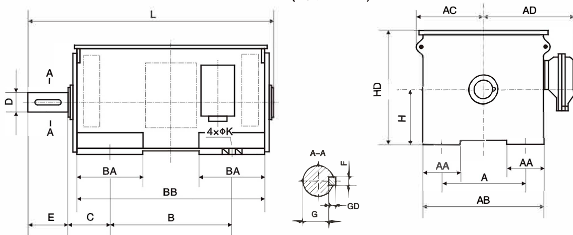
图3 Y500~630(4极及以上)
