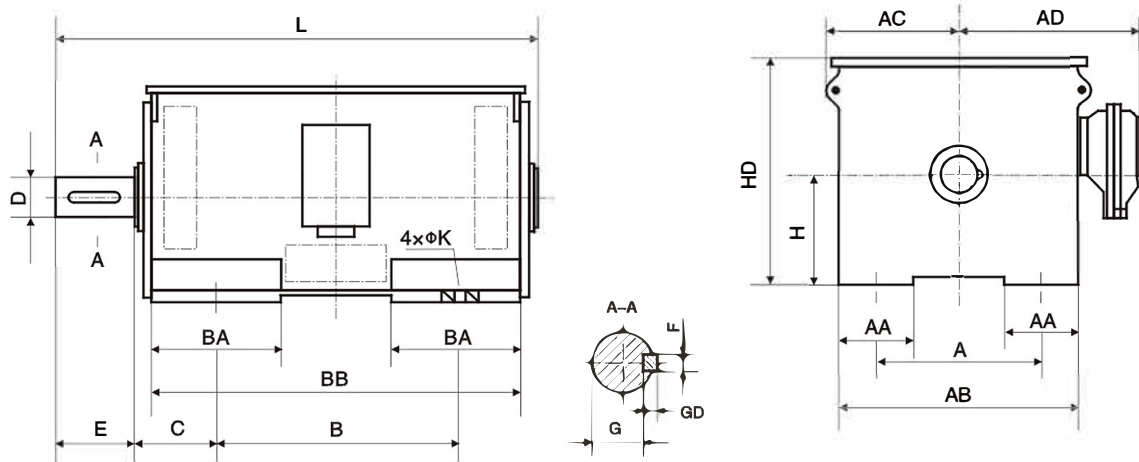
图2 Y400~450(4极及以上)
